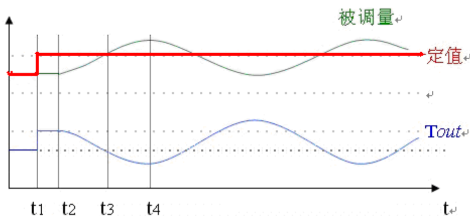
纯比例作用下的控制曲线图
