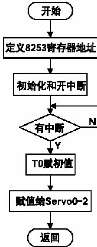
图4 基于8253产生PWA信号的软件流程
