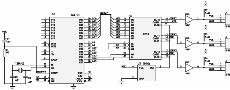
图 3 PWA 信号的计数和输出电路
