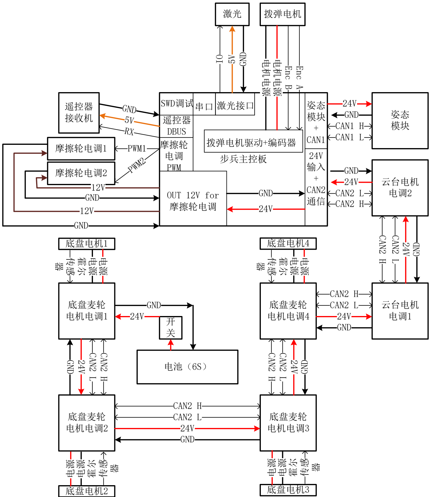
RM步兵电路框图
