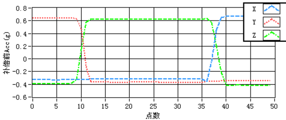
图 5-1 补偿前加速度计三轴静止+1g 输出
