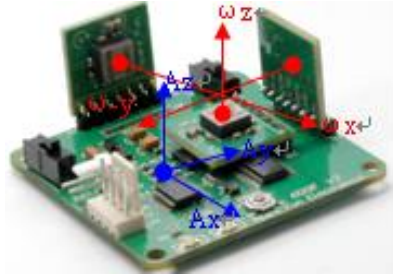
图 2-2 三轴陀螺仪和三轴加速度计组合
