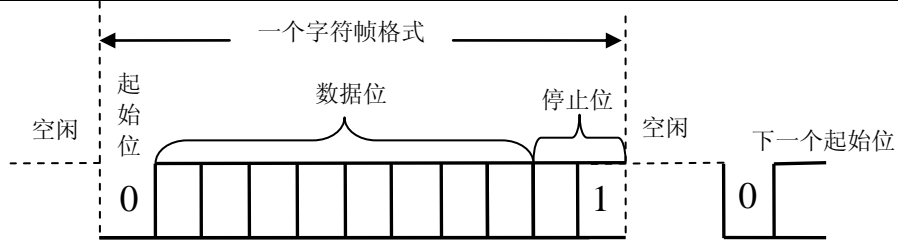
图 4-17 串口帧格式示意图
