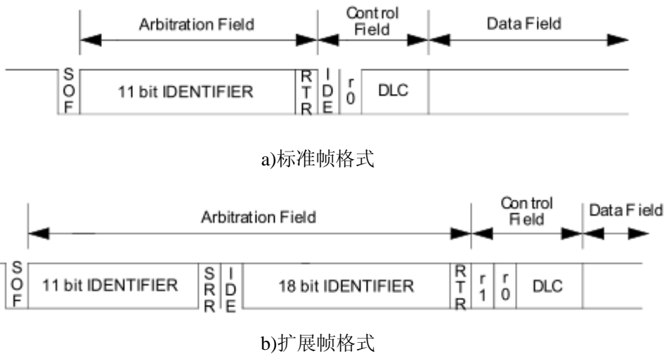
图 4-11 CAN 数据帧格式
