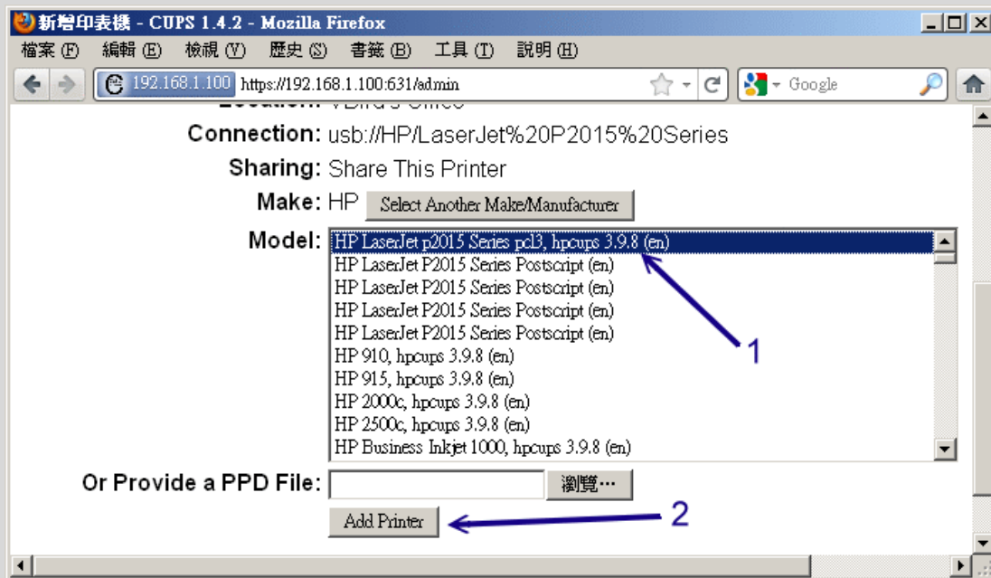
图 16.2-7、用 CUPS 设定 USB 打印机
