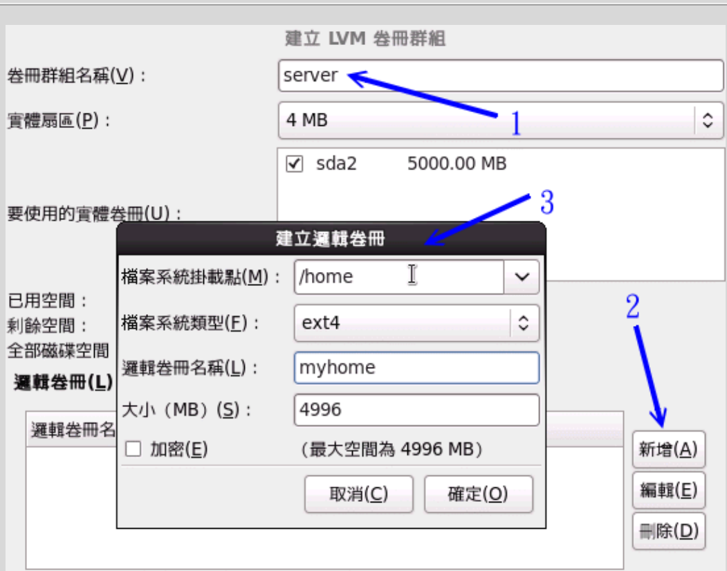
图 1.2-5、建立最终的 LVM 的 LV 与 /home
