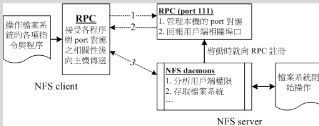
图 13.1-2、NFS 与 RPC 服务及文件系统操作的相关性
