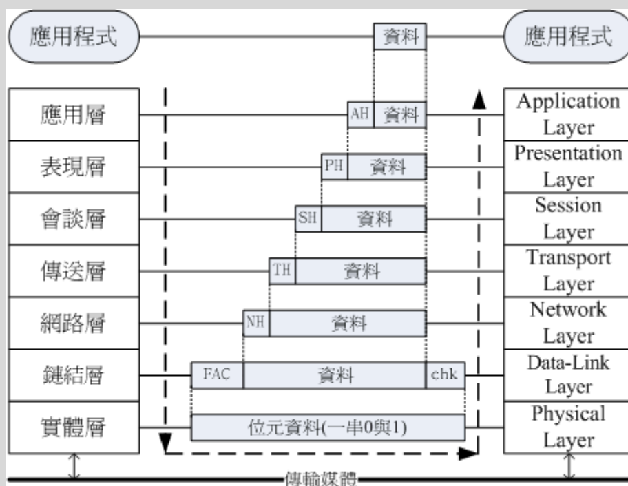
图 2.1-3、OSI 七层协议数据的传递方式
