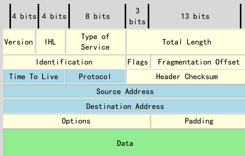
图 2.3-1、IP 封包的表头资料
